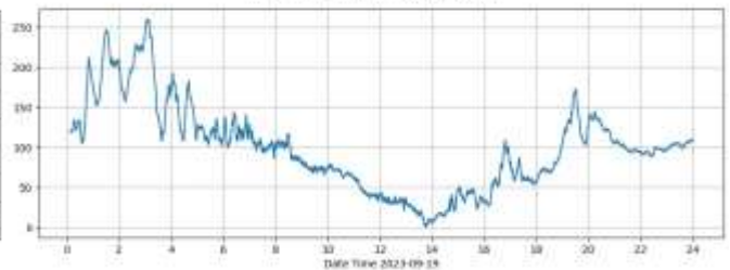
Wobister Magnetometer (59.17N, 3.06W)
