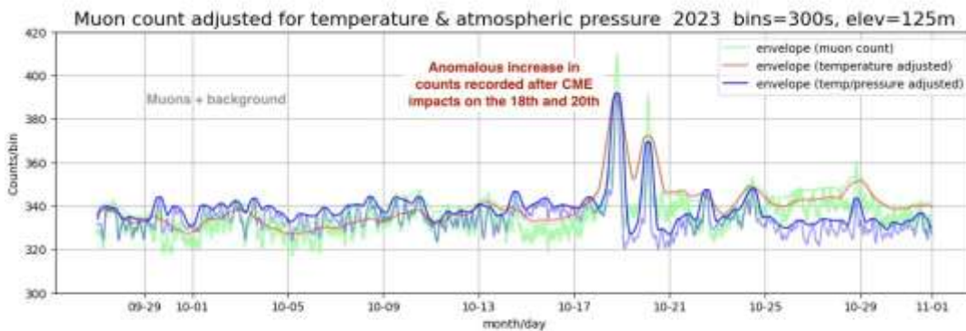
MUONS.
